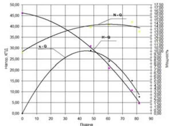
Рабочая характеристика ( \gamma=1000\text{кг/м}^3 , n=2900 об/мин)
