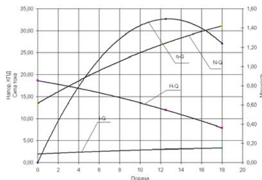
Рабочая характеристика ( \gamma=1000\text{кг/м}^3 , n=2900\text{ об/мин} )
