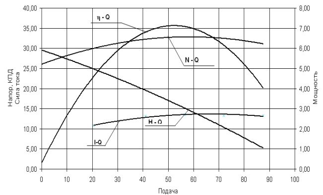
Рабочая характеристика ( \gamma=1000\text{кг/м}^3 , n=2900 об/мин)
