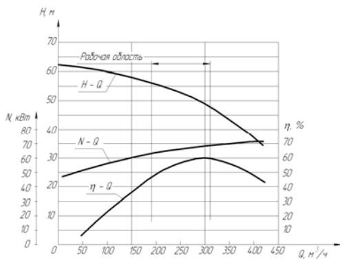
К 200-125-250Е - Б с двигателем 55кВт
