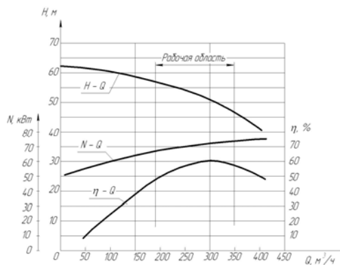
К 200-125-250Е с двигателем 75кВт
