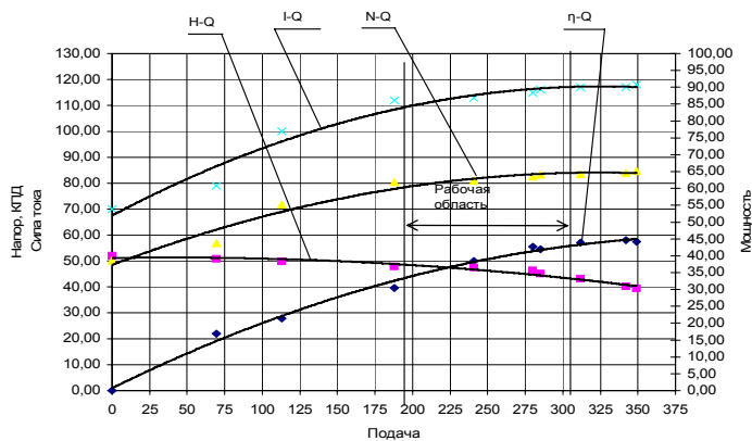
К 200-125-250Е с двигателем 55кВт
