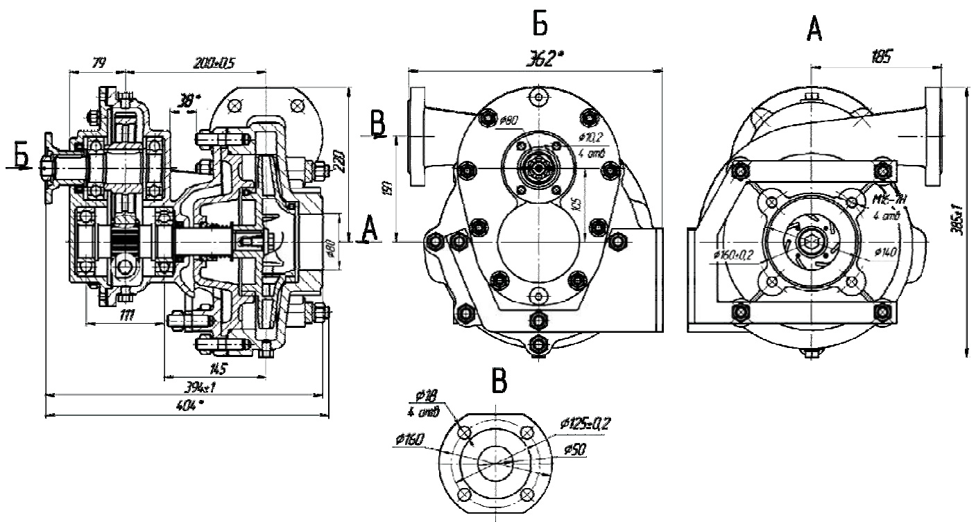
Габаритные и присоединительные размеры
